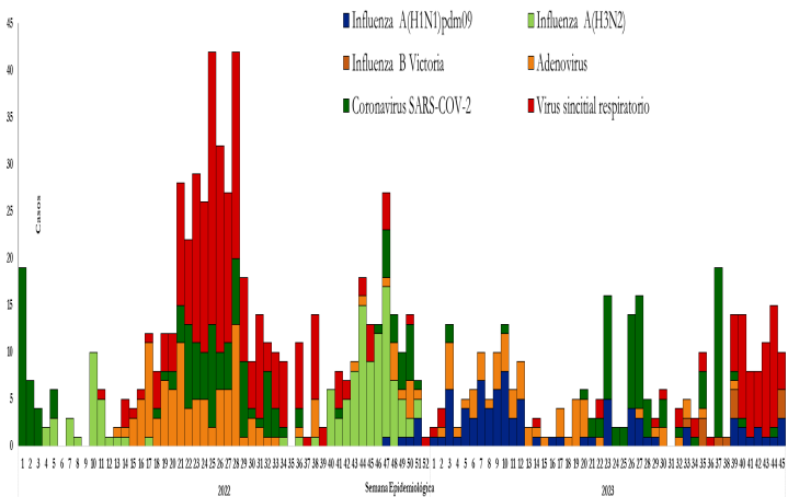
Fig.-5 Circulación de virus respiratorios desde la SE 1 de 2022 hasta la SE 45 de 2023 Vigilancia de sitios centinelas de influenza, República Dominicana
