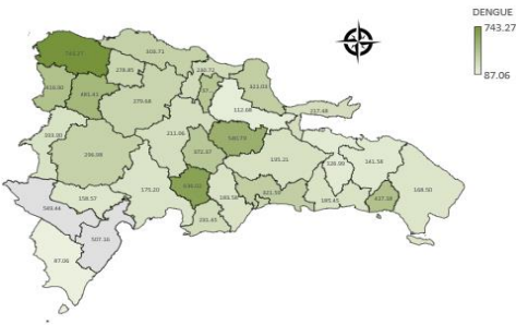
Fig.-2 Incidencia acumulada (por 100,000 hab.) de Dengue según provincia de residencia. SE 1-45, 2023. República Dominicana.
