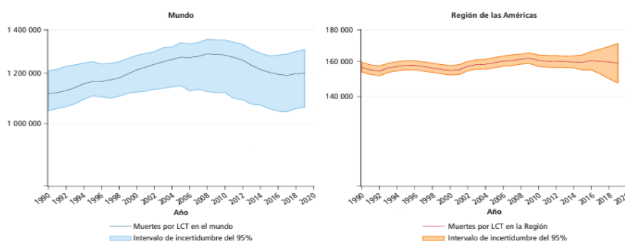
Fig.-1 Número de muertes en las vías de tránsito, 1990-2019
