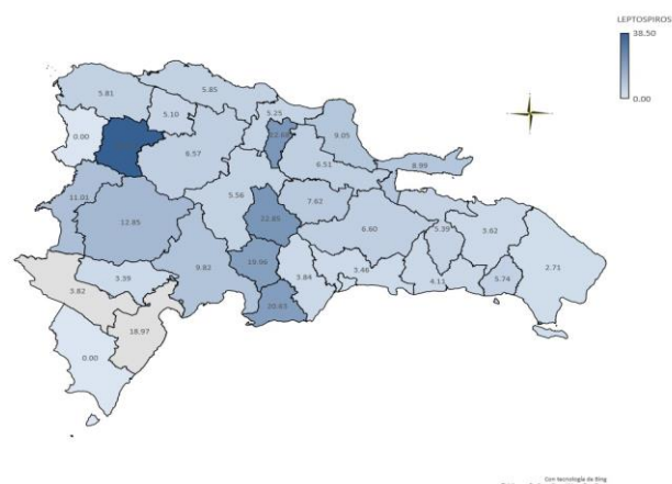
Fig.-4 Incidencia acumulada (por 100,000 hab.) de Leptospirosis según provincia de residencia. SE 1-45, 2023. República Dominicana.
